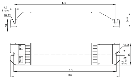
Рисунок 1 – Конвертер БАП40-1,0
